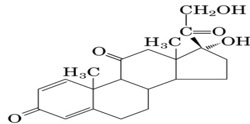
Prednisone
