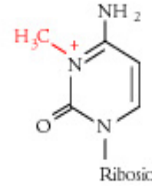
3-Metilcitosina ( m^3C )
