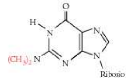
N^2,N^2 -Dimetilguanossina ( m^2G )
