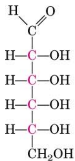
D-Allose
