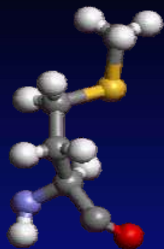
Met
