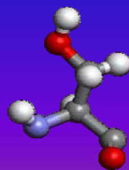
Ser
