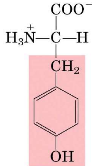
Tyrosine
