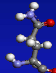
Gln
