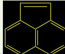
acenaftilene
