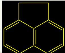
acenaftene
