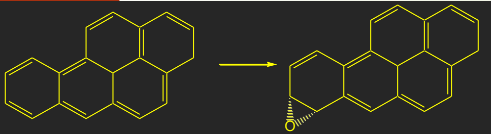
Benzo[a]piren-7,8-ossido
