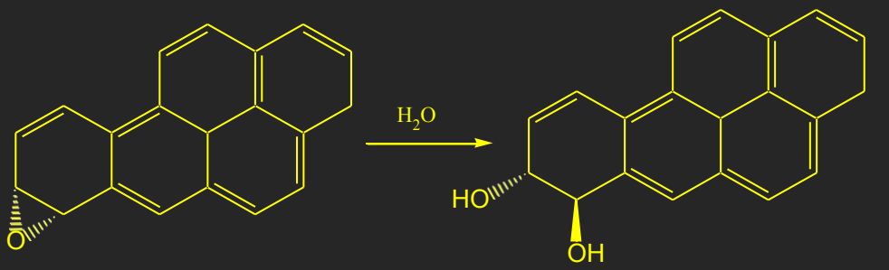
Benzo[a]piren-7,8-diidro-7,8-diolo
