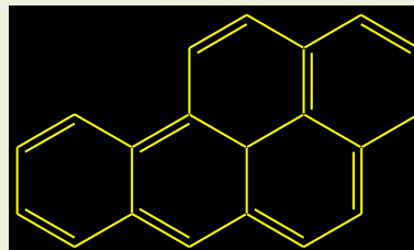
Benzo[a]pirene
