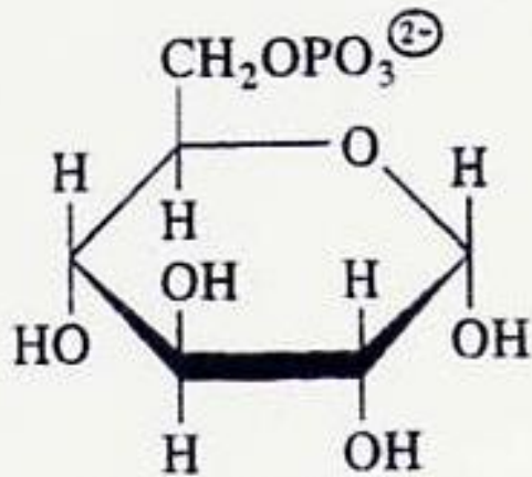
Glucosio 6-fosfato
