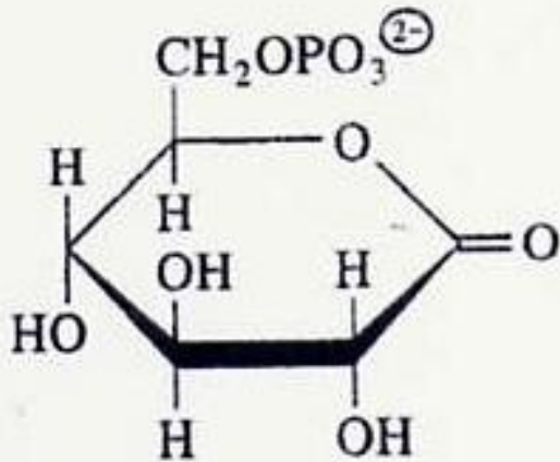
6-Fosfogluconolattone
