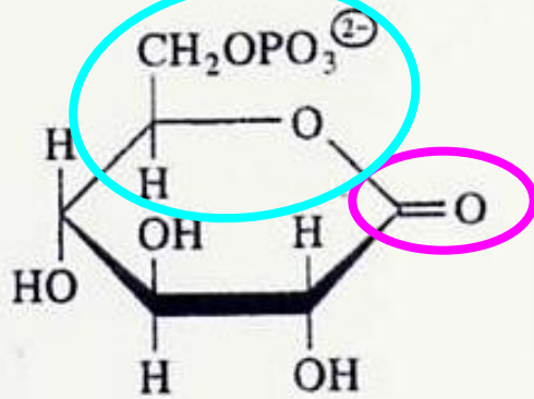
6-Fosfogluconolattone
