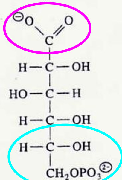
6-Fosfogluconato
