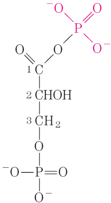
1,3-Bisfosfoglicerato
